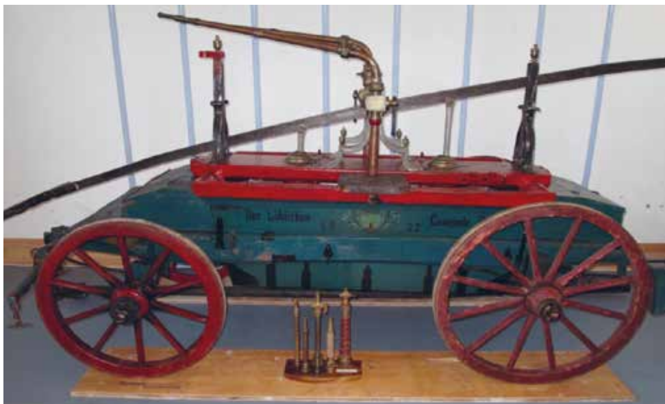
Fabrikat: Georg Huber, Schmid und Schlossermeister, 5627 Besenbüren Baujahr: 1822, Zylinder: 2, Dimensionen: Länge 4m, Breite 2m, Höhe 1,7m
